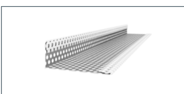
10. Cembrity Lüftungsprofil 0,6 mm perforierter Stahl, Länge 3000 mm
