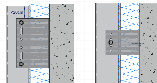
ÉQUERRE "POINT FIXE"
